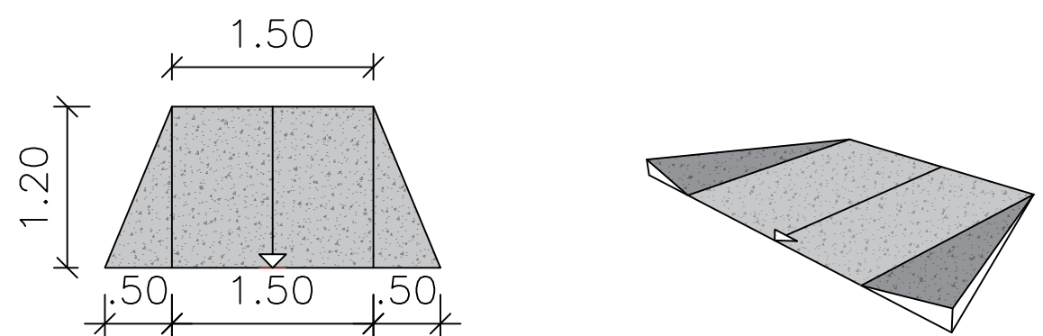
3 DETALHAMENTO DA RAMPA ACESSÍVEL ESCALA 1:50
