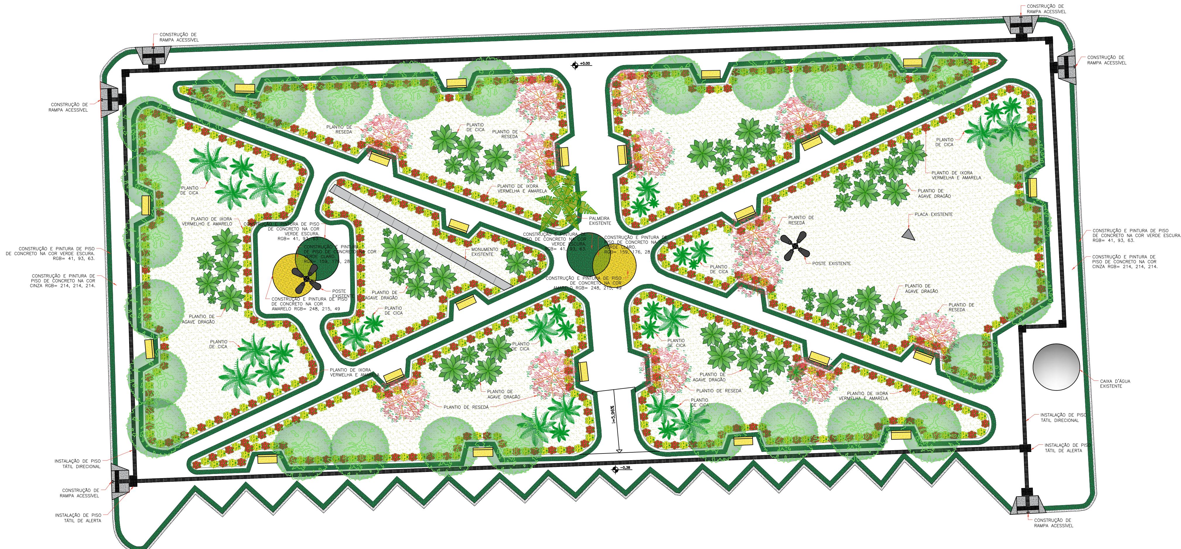
2 PLANTA DE CONSTRUÇÃO ESCALA 1:150
